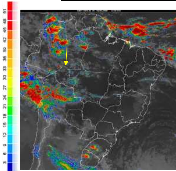
ig. 1- Mapa da precipitação de 04/05/2020: Imagem Góes canal IR topo das nuvens
