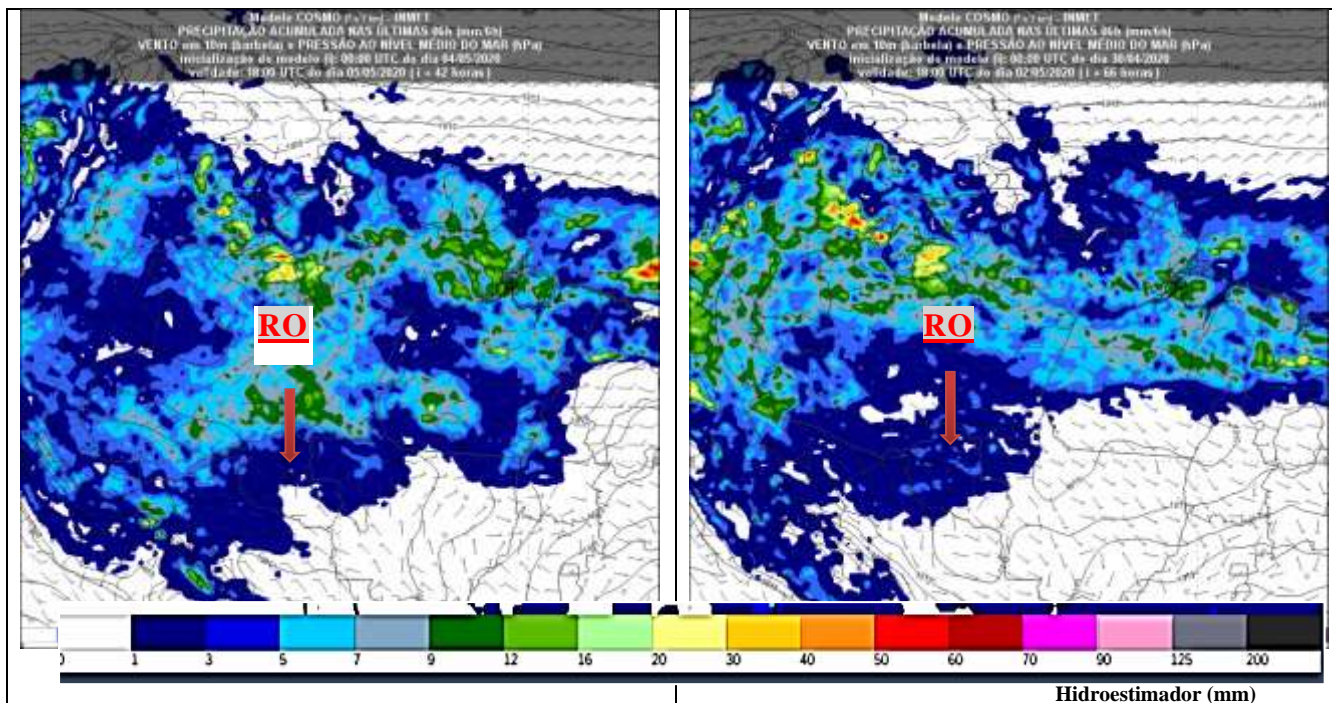
Fig.4 – Previsão de precipitação acumulada em RO, válida para 05/05/2020 18h Fonte: http://www.inmet.gov.br/ /
