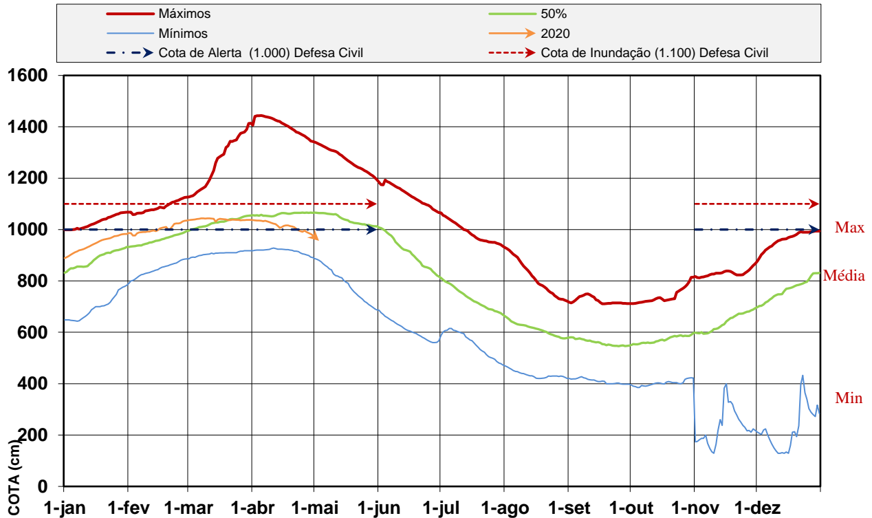
Gráfico 2- Monitoramento diário da cota do rio Mamoré, na coordenada geográfica de latitude 10,7925° leste e longitude 65,3478° oeste, município de Guajar-Mirim /RO - Srie histrica 1970 a 2017.
