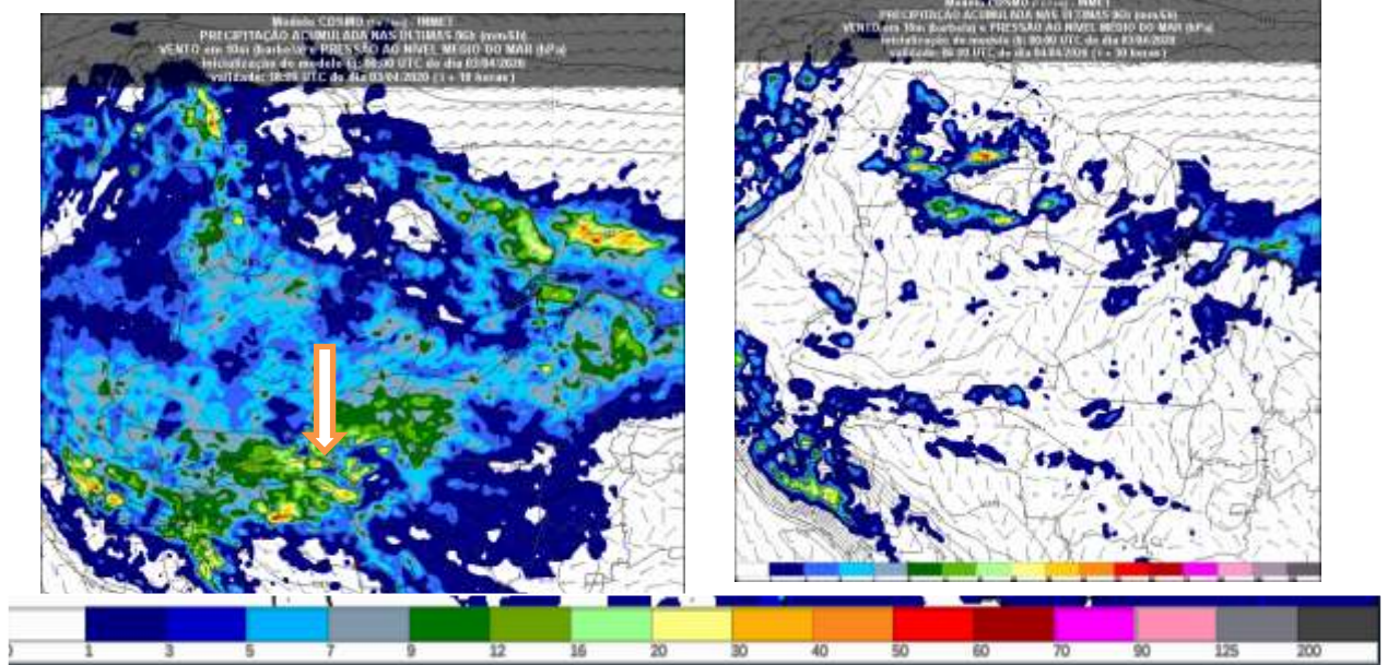
FIGURA 2 – Previsão do tempo no Estado de Rondônia para o dia 03/04/2020 as 18UTC
