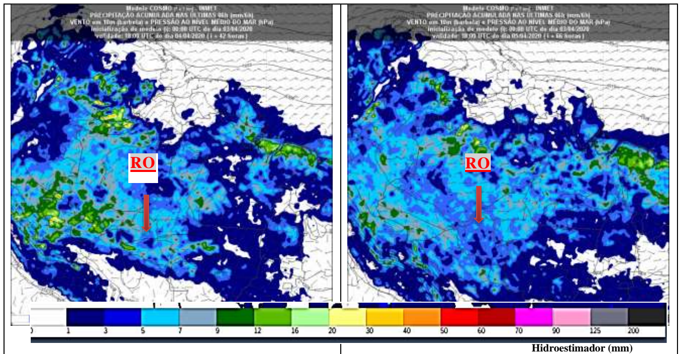
Fig.4 – Previsão de precipitação acumulada em RO, válida para 04/04/2020 18h Fonte: http://www.inmet.gov.br/
