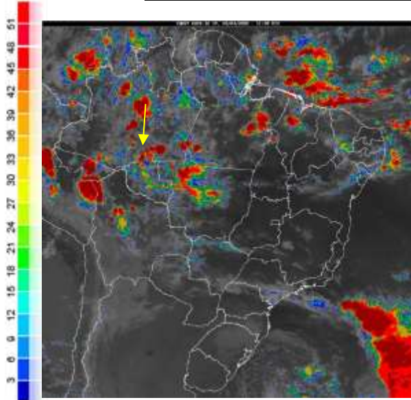
ig. 1- Mapa da precipitação de 30/03/2020: Imagem Góes canal IR topo das nuvens
