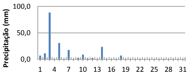
GRÁFICO 5.1 monitoramento da precipitação total diária, na estação pluviométrica Ariquemes, na ponte do rio Jamari, Br-421, em Ariquemes - RO.
