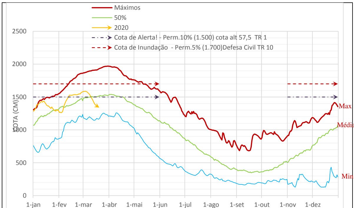
Gráfico 3 - Monitoramento diário da cota do rio Madeira, na coordenada geográfica de latitude -8,7483 leste longitude -63,9169 oeste, Ponte Br-319, Porto Velho/RO.
